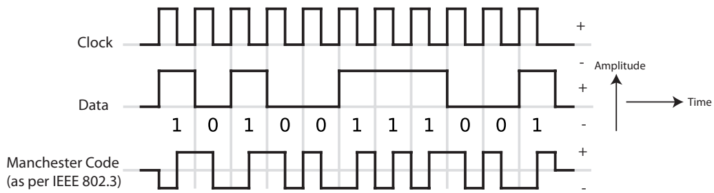
(Fig. 2, Manchester Code)
